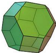
Усечённый октаэдр (24, 36, 14)
