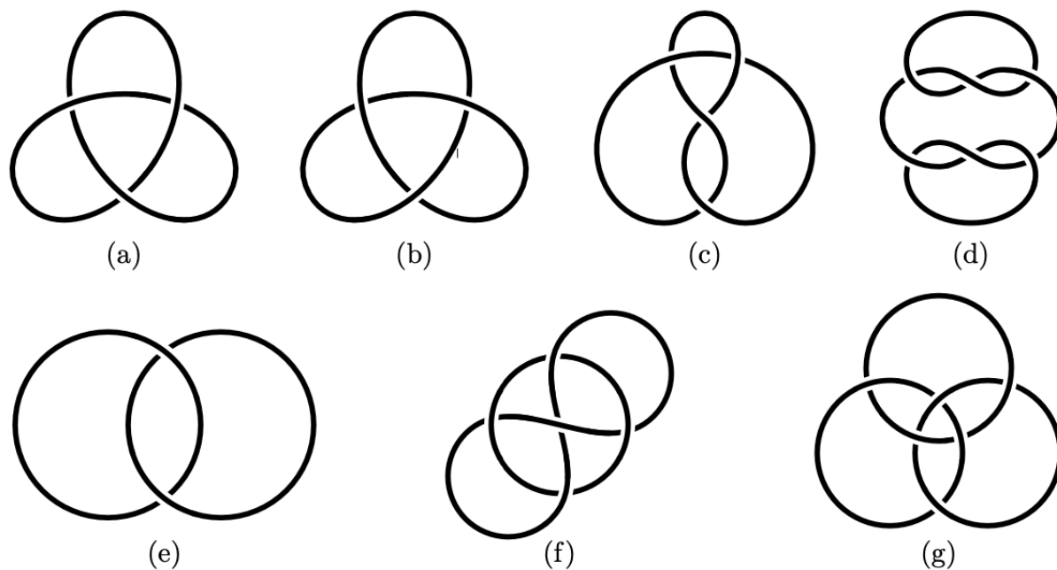
РИС. 1. а) правый трилистник; б) левый трилистник; с) восьмёрка; d) бабушкин узел; е зацепление Хопфа; f) зацепление Уайтхеда; g) кольца Борромео.
