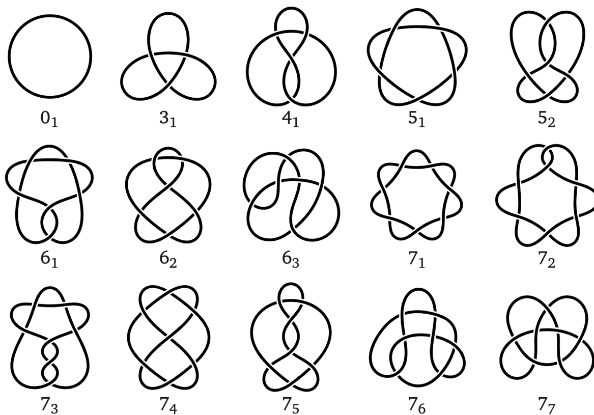
РИС. 2. Все узлы с \leq 7 перекрёстками.
