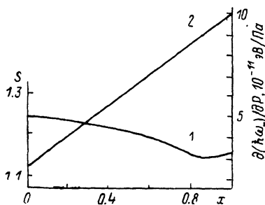
Рис. 2. Зависимость от состава x параметров S (1) и d(\hbar\omega_r)/dP (2).
