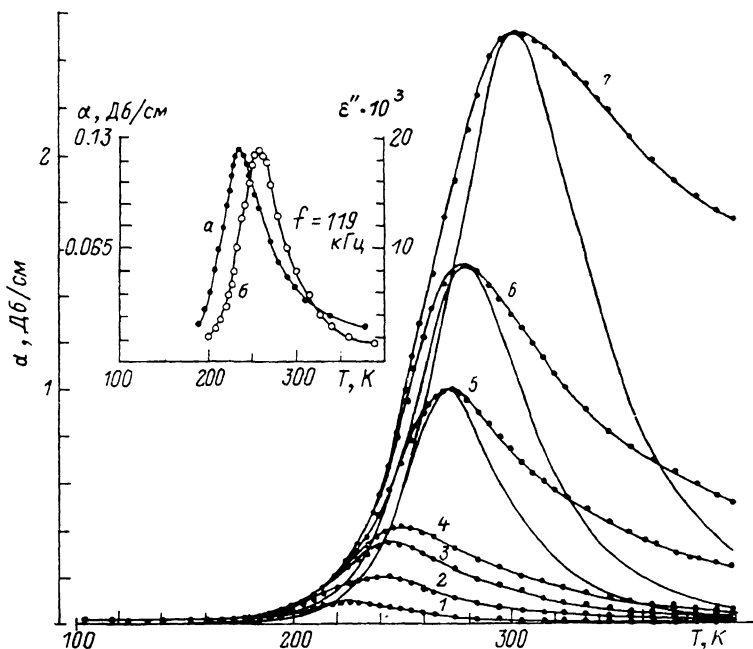
Рис. 1. Температурная зависимость поглощения ультразвука \alpha(T) (а) и диэлектрической проницаемости \epsilon''(T) (б) в монокристаллах \alpha-LiIO_3 (рН=2).
