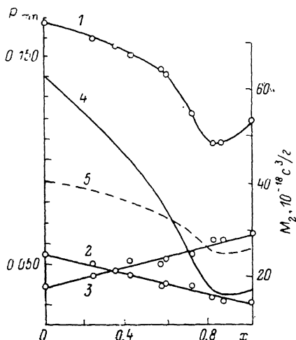
Рис. 1. Зависимость от состава x коэффициентов P_{11} (1), P_{12} (2), P_{44} (3), M_2 (4). \lambda_0=1.15 мкм.
