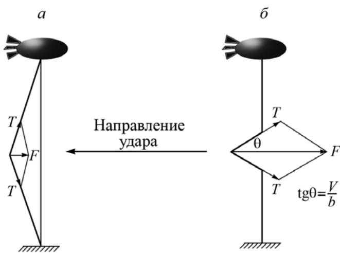
Схема сил, возникающих при квазистатическом (а) и динамическом (б) отклонениях троса при ударе
