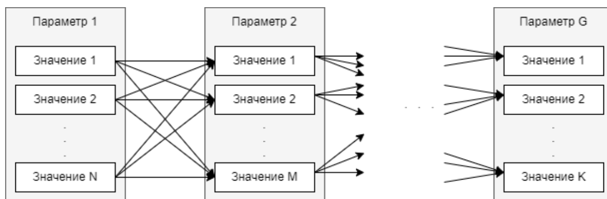
Рис 5. Структура графа для решения дискретной параметрической задачи
