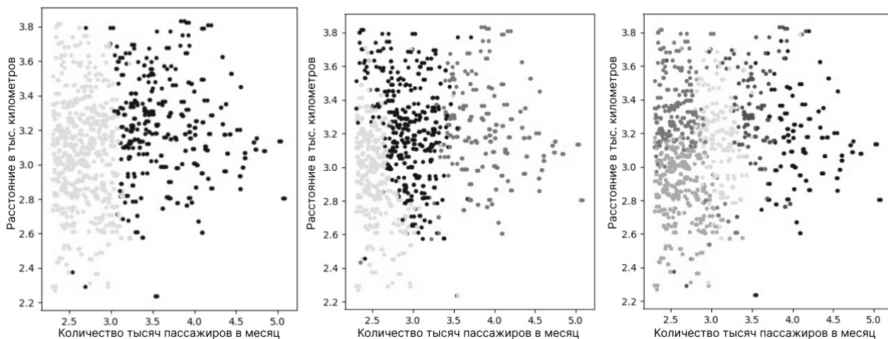
Рис 4. Примеры кластеризации пассажирских авиационных маршрутов на 2, 3 и 5 кластеров
