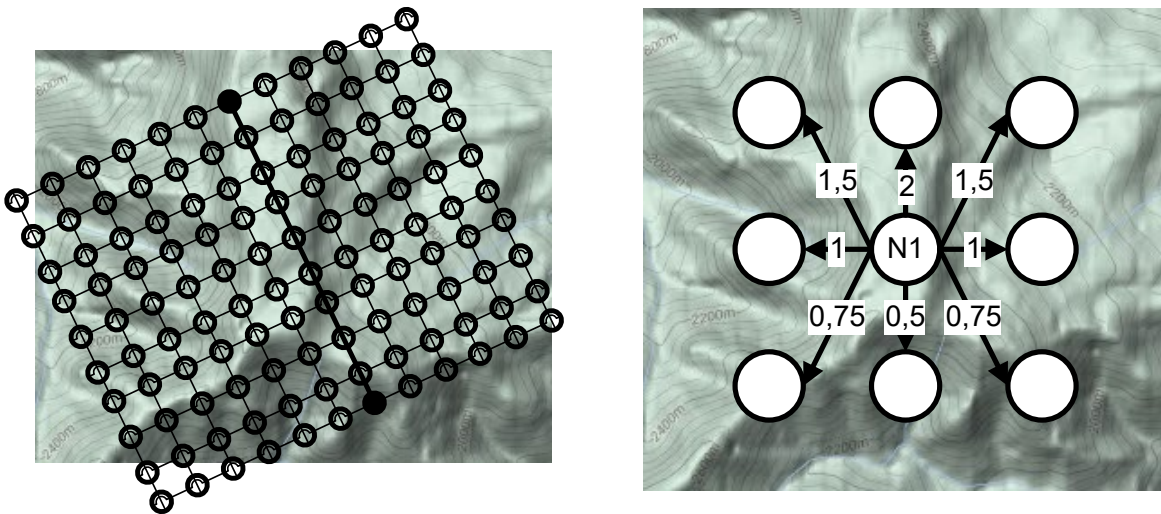
Рис 2. Пример построения маршрута по координатной сетке на местности (слева) и пример построения дуг из вершины N1 в соседние вершины сетки и установка весов слоя H при условии целевой вершины сверху вершины N1 (справа)
