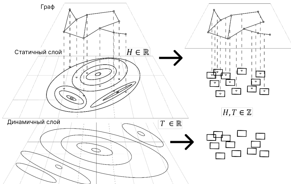
Рис 1. Разделение информации о графе на слои в методе муравьиных колоний
