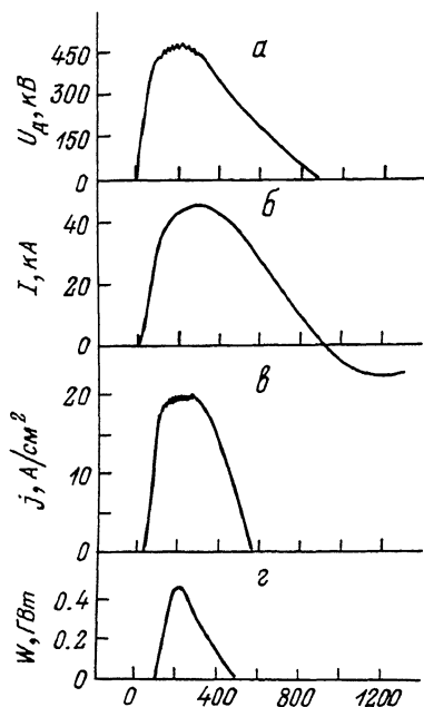
Рис. 1. Осциллограммы импульсов ускоряющего напряжения (а), тока в диоде (б), плотности электронного тока за фольгой (в) и лазерного излучения (г) при зарядном напряжении 80 кВ.
