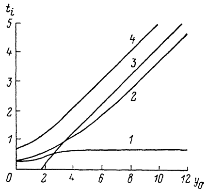
Рис. 2. Зависимости характерных моментов времени динамики ФД от начальной оптической толщины слоя y_0 = \sigma_B L N_0 .
