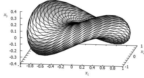
Рис. 1. Неголономная геодезическая сфера.
