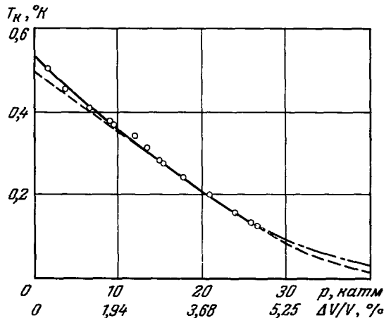
Рис. 23. Зависимость температуры сверхпроводящего перехода кадмия от давления и относительного изменения объема.
