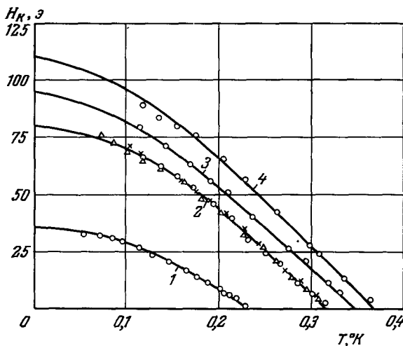
Рис. 26. Кривые критических полей титана. Кривые: 1 — p = 1 атм; 2 — \circ — p = 15500 атм, \times — 900 атм, \Delta — 9200 атм; 3 — p = 18400 атм; 4 — p = 24400 атм.
