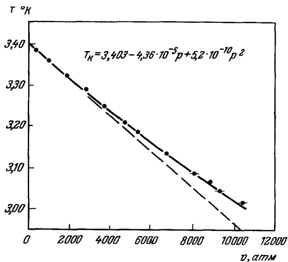
Рис. 10. Изменение температуры сверхпроводящего перехода индия при сжатии.
