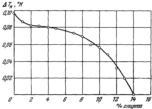
Рис. 1. Зависимость давления в бомбе постоянного объема при температуре жидкого гелия от концентрации спирта-сырца в водно-спиртовом растворе. По оси ординат отложено изменение температуры сверхпроводящего перехода олова \Delta T_k = (T_k)_{p=0} - T_k(p) ; \Delta T_k = -4,5 \cdot 10^{-5} p ( p — в атм), так что \Delta T_k = 0,1^\circ \text{K} соответствует p \approx 2000 атм.
