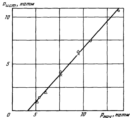
Рис. 3. Зависимость давления в бомбе при температуре ниже 77° К от давления при комнатной температуре.
