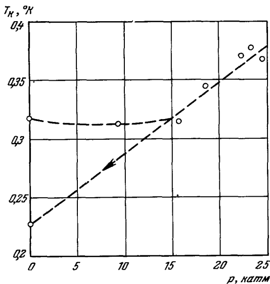
Рис. 28. Зависимость температуры сверхпроводящего перехода титана от давления.
