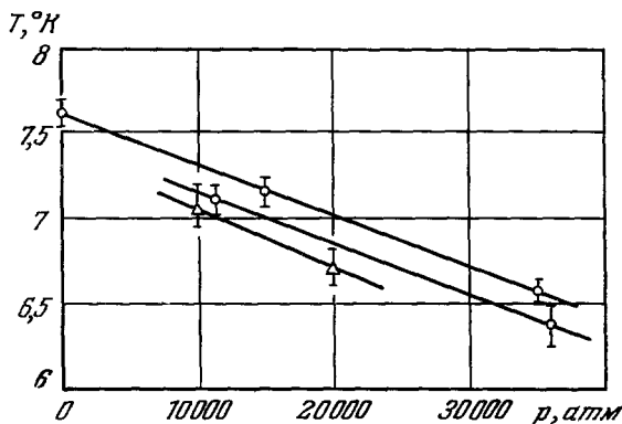
Рис. 35. Зависимость температуры сверхпроводящего перехода Ga\ II от давления.
