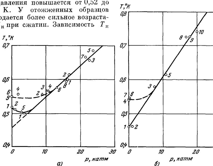
Рис. 27. Зависимость температуры сверхпроводящего перехода от давления.
