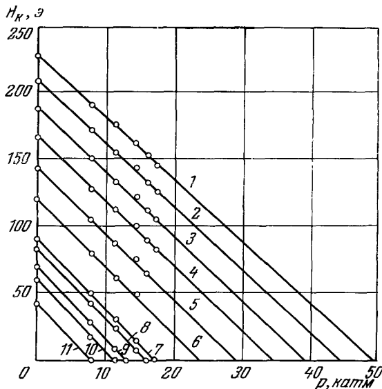
Рис. 14. Зависимость критического поля индия от давления.
