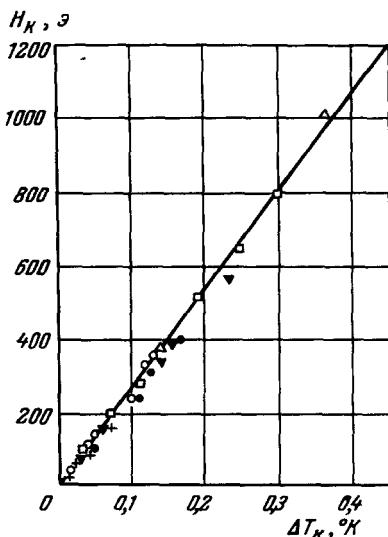
Рис. 31. Критические поля Bi III при давлениях:
