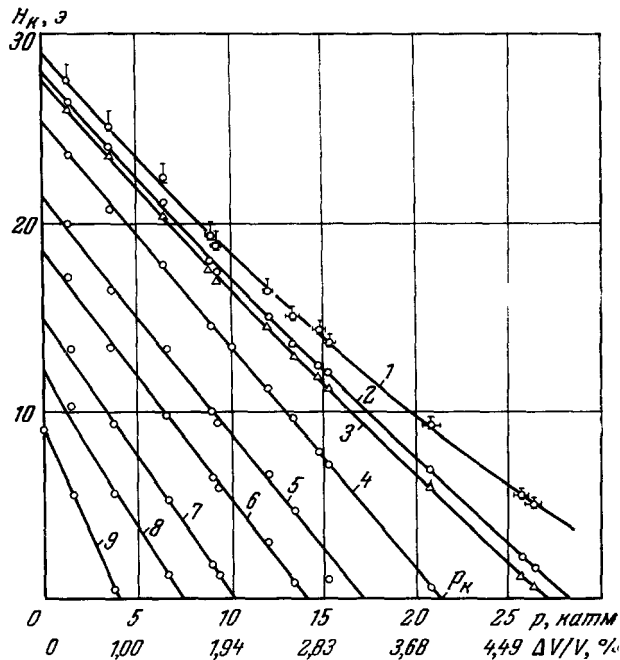
Рис. 24. Зависимость критического поля кадмия от давления и относительного изменения объема.
