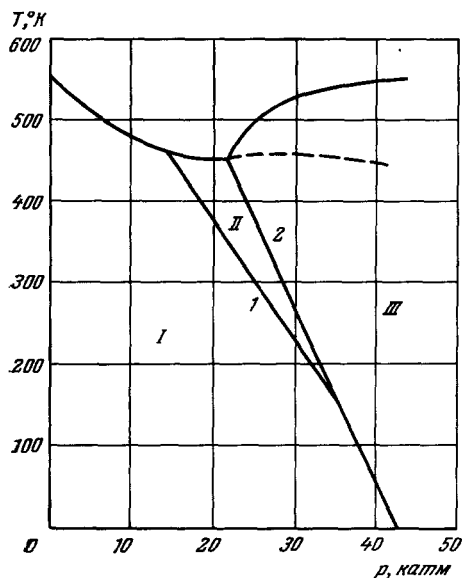
Рис. 29. Фазовая диаграмма висмута.
