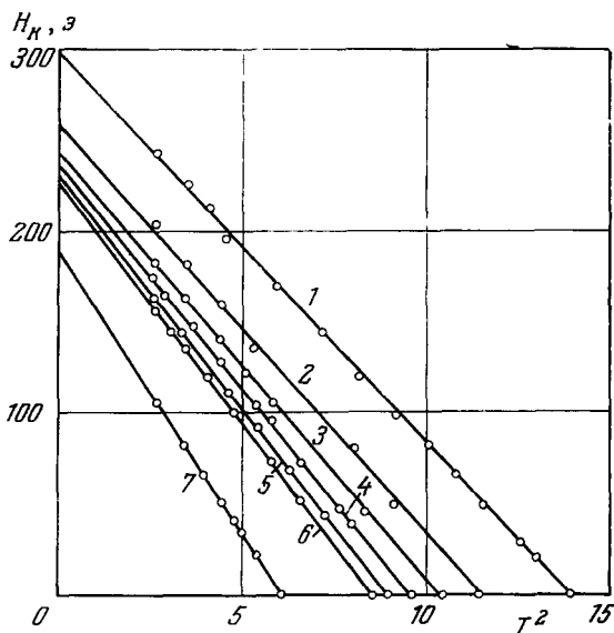
Рис. 11. Кривые критических полей для олова при различных давлениях.
