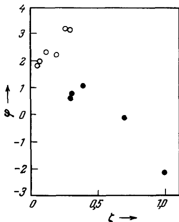
Рис. 37. Экспериментальные значения \varphi = \frac{\partial \ln NV}{\partial \ln v} как функция \zeta .
