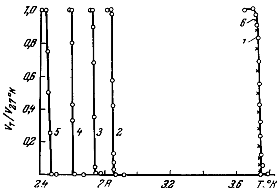
Рис. 5. Кривые сверхпроводящего перехода оловянного манометра при различных давлениях, p (атм): 1 — 0; 2 — 19 750; 3 — 22 000; 4 — 25 000, 5 — 28 400; 6 — давление снято. По оси ординат отложено относительное изменение сигнала на выходе радиотехнической установки.
