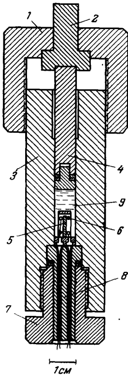
Рис. 2. Бомба высокого давления.
