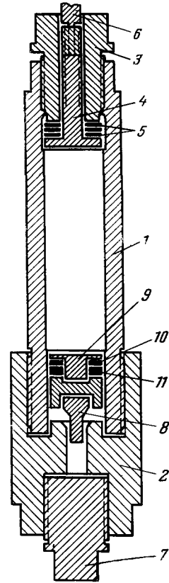
Рис. 4. Мультипликатор.
