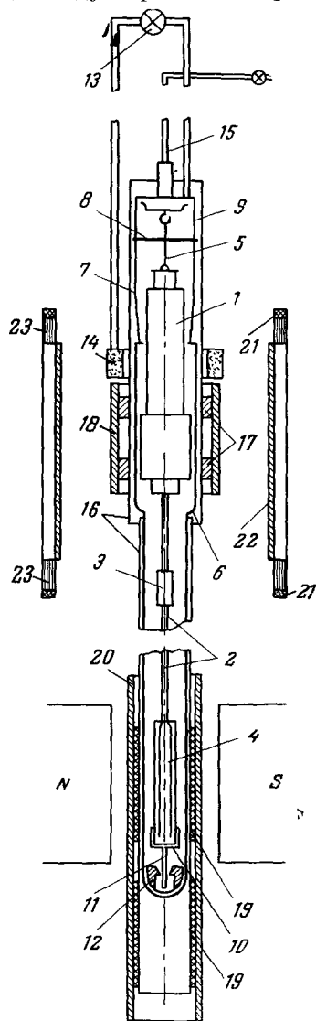
Рис. 6. Схема прибора для исследования сверхпроводящих свойств металлов при высоких давлениях в области сверхнизких температур.
