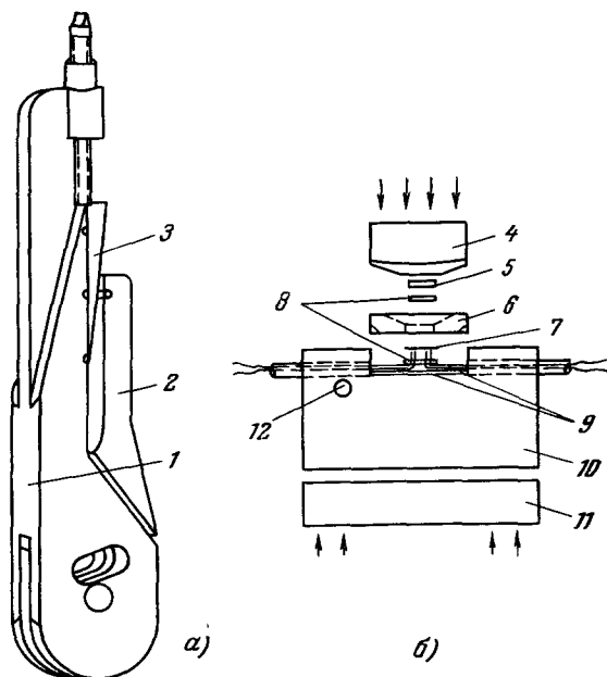
Рис. 8. а) Регулируемый низкотемпературный зажим: 1 — корпус; 2 — подвижный рычаг; 3 — клин; б) камера высокого давления: 4 — поршень; 5 — бронзовая прокладка; 6 — держатель образца; 7 — образец; 8 — верхняя и нижняя стеатитовые шайбы; 9 — слюдяные прокладки; 10, 11 — опорные подложки; 12 — угольный термометр.
