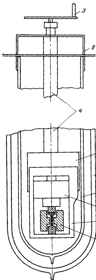
Рис. 7. Схема низкотемпературного пресса.
