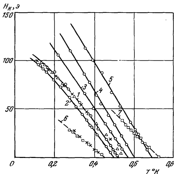
Рис. 25. Кривые критических полей циркония у образцов неотожженных (сплошные кривые) и отожженных (пунктир).
