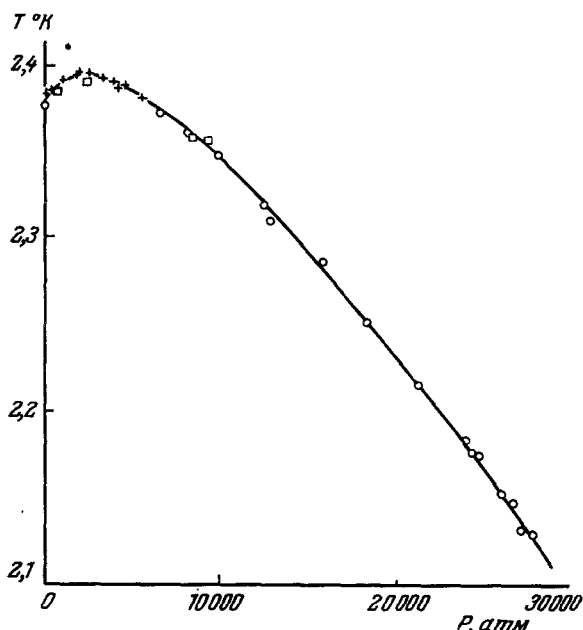
Рис. 20. Зависимость температуры сверхпроводящего перехода таллия от давления по данным различных авторов.
