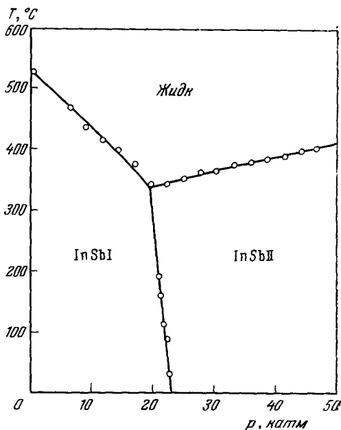
Рис. 33. Фазовая диаграмма InSb.
