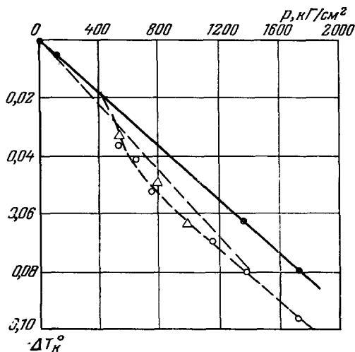
Рис. 15. Зависимость \Delta T_K от p для индия (сплошная кривая) и для олова (пунктирные кривые).
