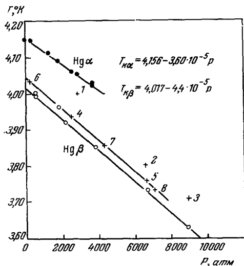
Рис. 18. Зависимость критической температуры от давления для двух модификаций ртути.
