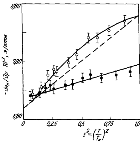
Рис. 19. Зависимость \partial H_K/\partial p от приведенной температуры для \alpha - и \beta -модификаций ртути.
