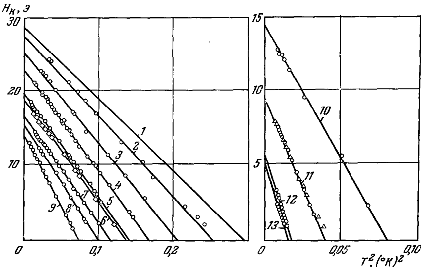
Рис. 22. Зависимость критических полей кадмия от температуры.
