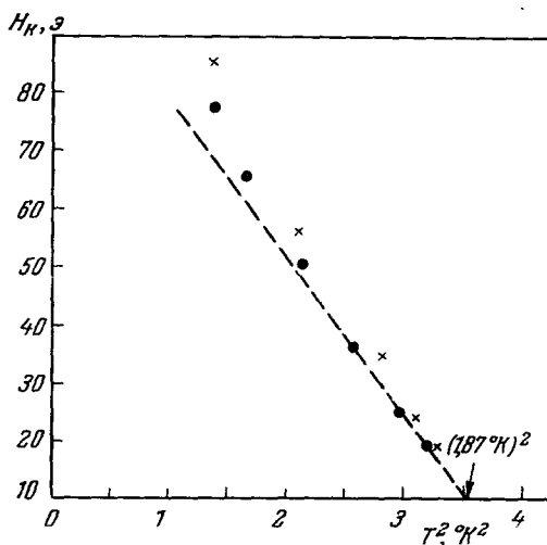
Рис. 34. Критические поля InSb II. \times и \bullet — различные образцы InSb (I и II).
