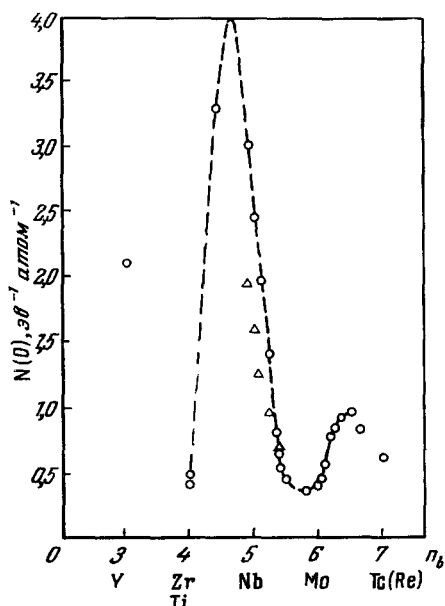
Рис. 38. Зависимость плотности состояний N(0) от числа валентных электронов.
