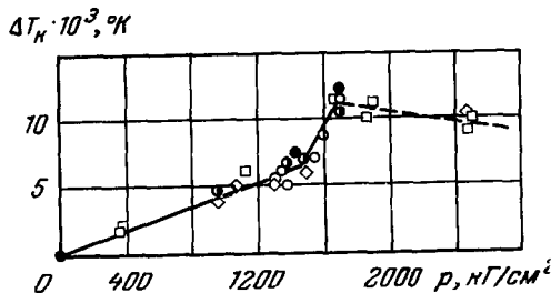
Рис. 21. Зависимость смещения температуры сверхпроводящего перехода от давления для таллия.
