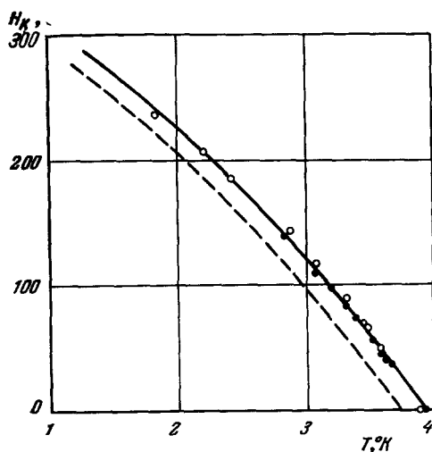
Рис. 30. Критические поля Bi II. ○ — p = 26\,400 \text{ атм} ; ● — опыт без оловянного манометра. Пунктиром изображена кривая критических полей для олова.
