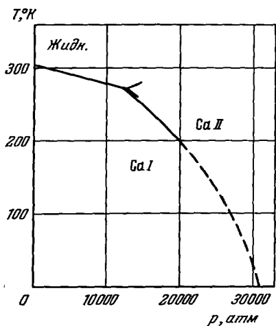
Рис. 32. Фазовая диаграмма галлия.
