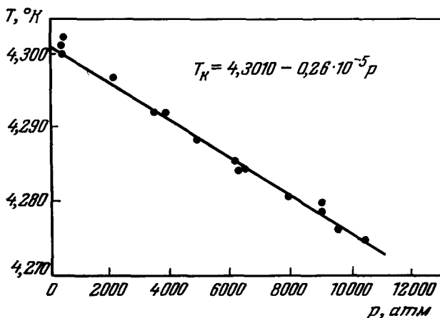
Рис. 16. Зависимость температуры сверхпроводящего перехода от давления для образца тантала, отожженного при температуре 2300° С.
