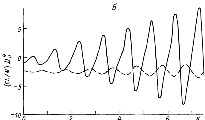
Рис. 1. Характеристики биконического участка, на котором возбуждаются HE_{11} - и HE_{12} -моды. Показатель преломления цилиндрической однородной перегайки радиусов b - n_1 = 1.45 , внешней среды - n_2 = 1.0 . а - зависимость |\eta| - пунктирная кривая, \beta_R и E = \frac{2c|\eta|\beta_R}{\omega} - сплошные кривые от нормированной частоты
