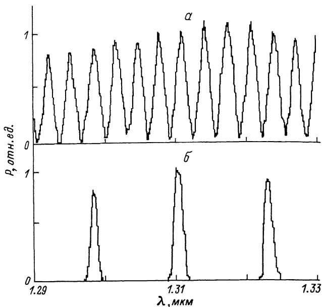
Рис. 3. Спектры пропускания. а - биконическая неоднородность с N = 400 ; б - четыре последовательные биконические неоднородности с N_1 = 1.33 \cdot N_2 = 2 \cdot N_3 = 4 \cdot N_4 = 400 и \Delta_4 = 2\Delta_3 = 3\Delta_2 = 4\Delta_1 = 6.5 нм, разделенные участками ОВС, поглощающими высшие моды.
