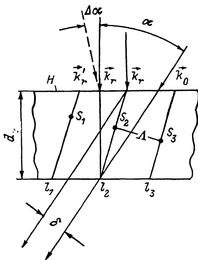
Рис. 1. К рассмотрению угловой и спектральной селективности глубокой трехмерной голограммы.
