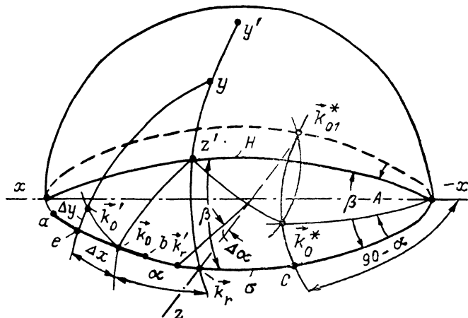
Рис. 2. К рассмотрению направления распространения сопряженной волны и угловой селективности излучения, восстановленного псевдоглубокой голограммой.
