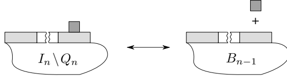
Рис. 17. К лемме 4
