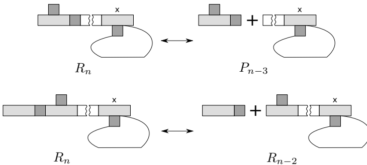
Рис. 19. К лемме 6
