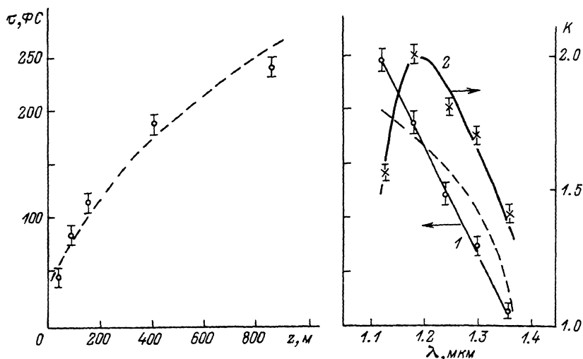
Рис. 2. а) Зависимость длительности ЦП АКФ \tau от длины световода ( \lambda=1.18 мкм). Штриховая линия - теоретическая зависимость (4). б) Зависимость длительности ЦП АКФ \tau и контраста АКФ K от длины волны в ОВС длиной 400 м. Штриховая линия - теоретическая зависимость (4).
