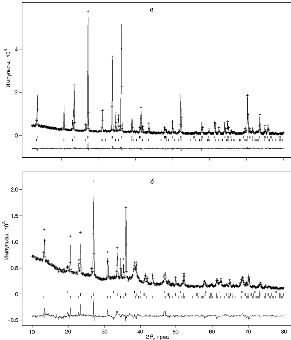
Рис. 2. Результат анализа методом Ритвелда исходного порошка \text{Si}_3\text{N}_4 (а) и образца \text{Si}_3\text{N}_4/\text{KBr} 10/90 (б), сохраненного после нагружения до 36 ГПа:
