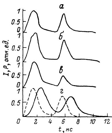
Рис. 1. Осциллограммы импульсов.
