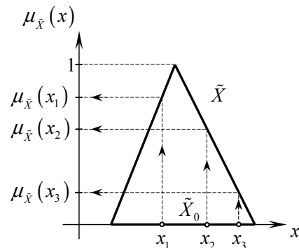
Рис. 5. Пример выпуклой функции принадлежности
