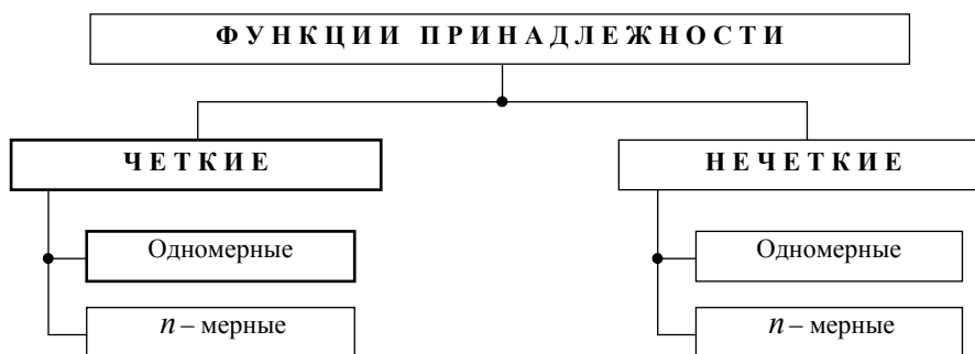
Рис. 1. Обобщенная классификация функций принадлежности
