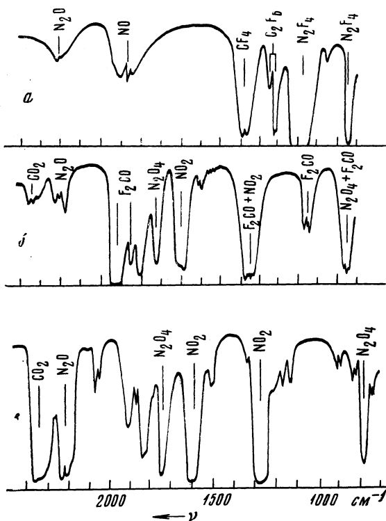
Рис. 1. Инфракрасные спектры поглощения. a — исходная смесь: N_2F_4 (100 тор), NO (200 тор) CF_4 , C_2F_6 ; b — смесь после облучения, опыт 5, NO_2 , F_2CO ; c — смесь после облучения, опыт 6, NO_2 , CO_2 , N_2O
