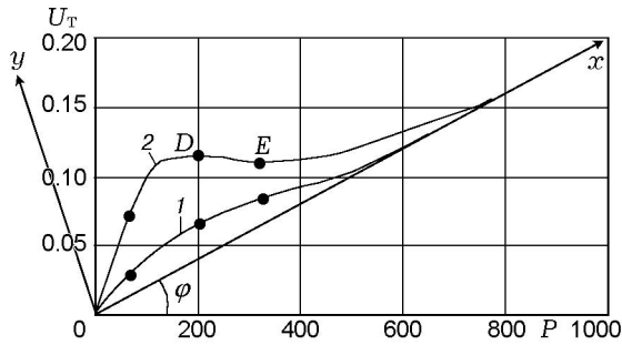
Рис. 2. Экспериментальные зависимости U_T(P) :
