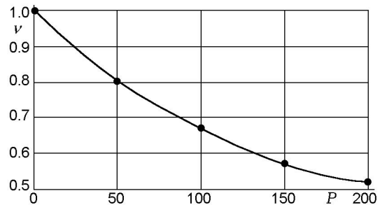
Рис. 4. Изменение показателя степени \nu как функции давления для кривой 1 на рис. 2
