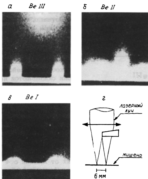
Рис. 1. Схема эксперимента (г) и спектрограммы факелов в излучении на переходах ионов Be I-III (а-в).
