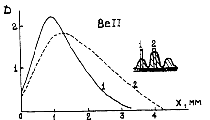
Рис. 2. Относительные интенсивности свечения лазерного факела (1) и области взаимодействия (2) на переходах ионов \text{BeII} , \text{III} .
